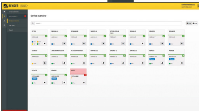
Darstellung von Gerätedaten auf der Weboberfläche (COM465IP)
