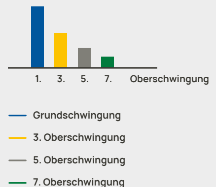
Oberschwingungsspektrum
